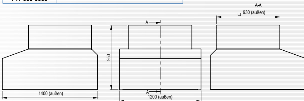
Angeschraubt am Domschachtkragen
