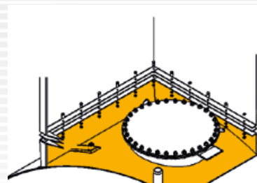
Angeschraubt am Domschachtkragen
